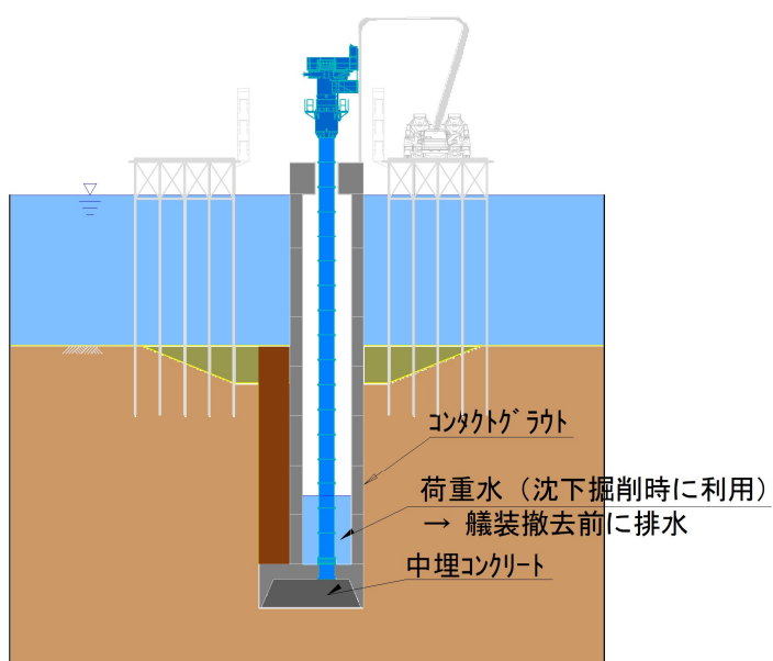
中埋コンクリート打設状況（作業室内）
